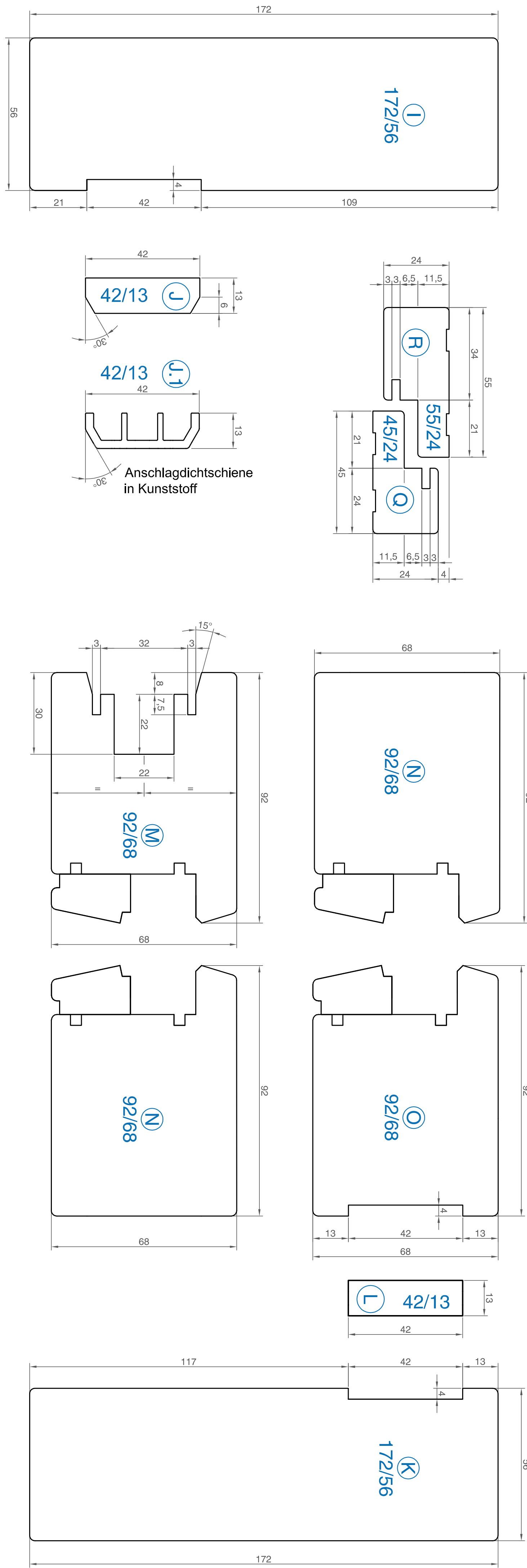
Elemente GFK M 1:1
